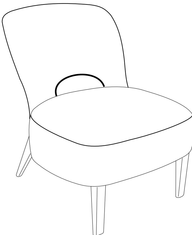
Moon
